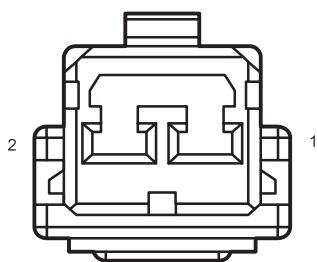
D20 Left Rear Door Tweeter
