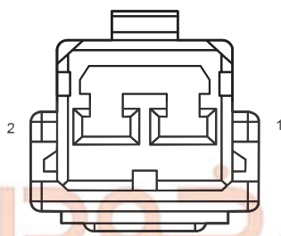
D13 Right Front Tweeter
